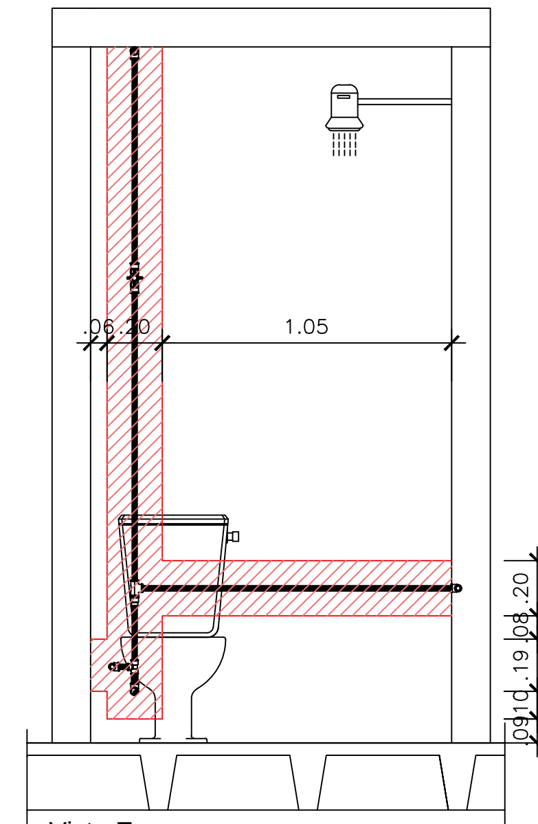
Vista E ESCALA 1/25
