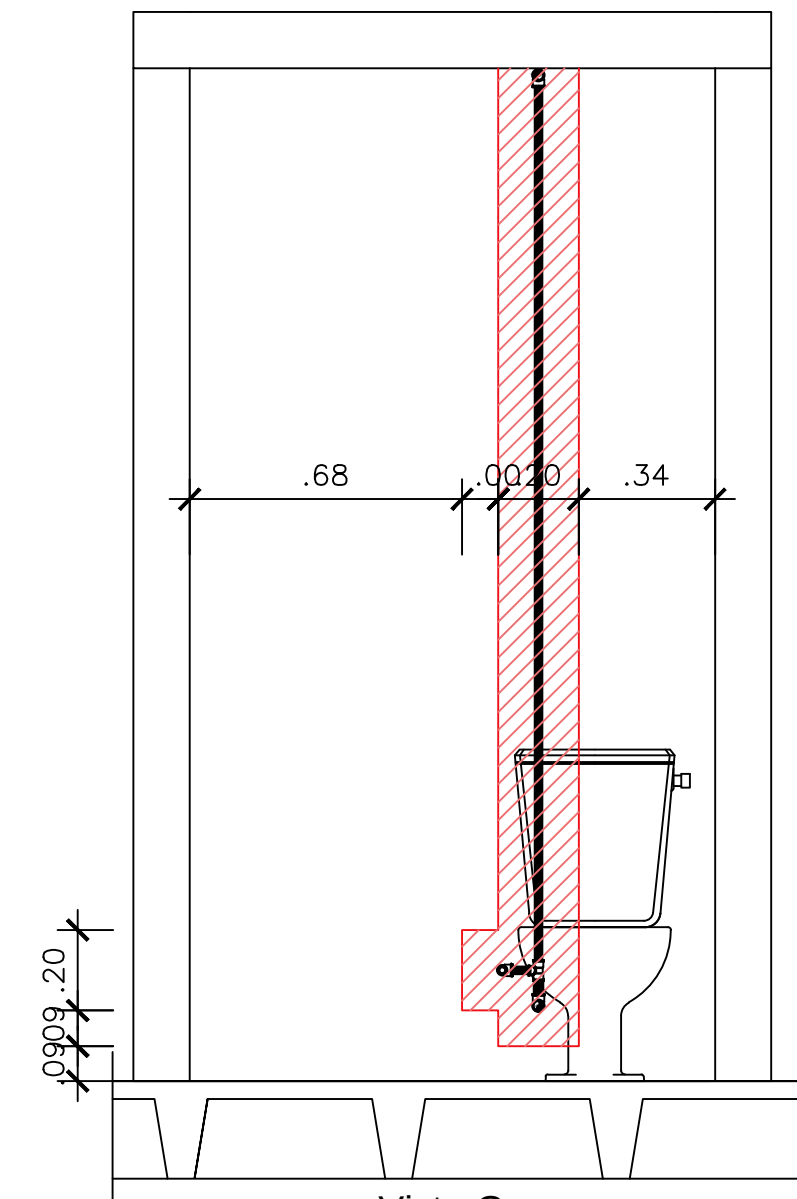
Vista G ESCALA 1/25
